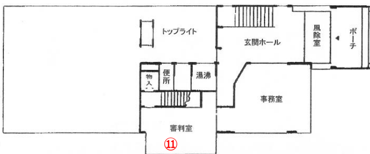
1階平面図(214.24㎡)
